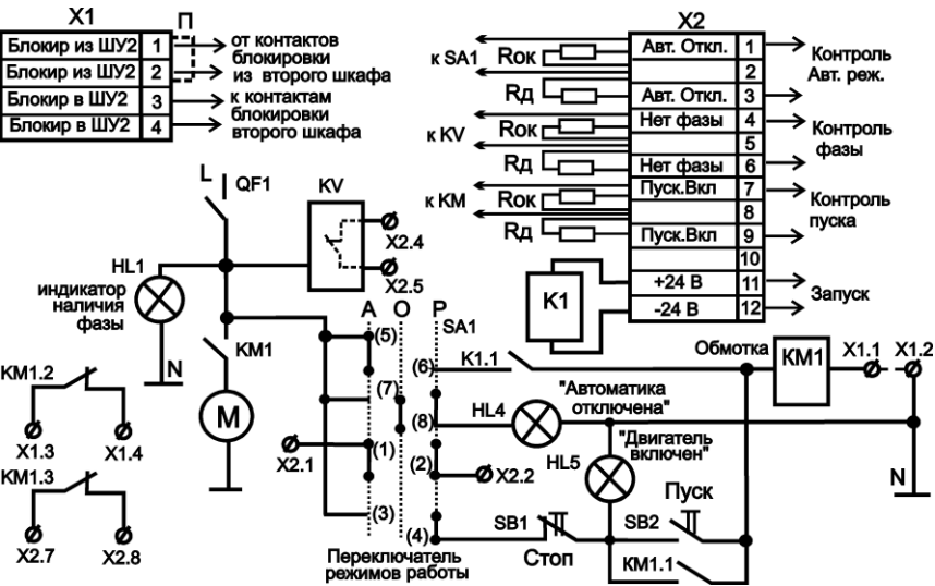
Рис. 1 - Схема ШУ с рабочим напряжением 220 В
