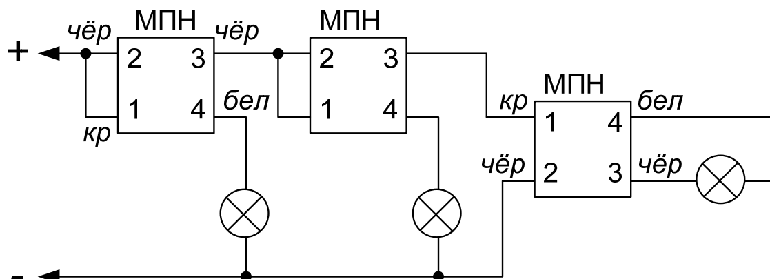
Подключение нескольких оповещателей к одному выходу прибора
