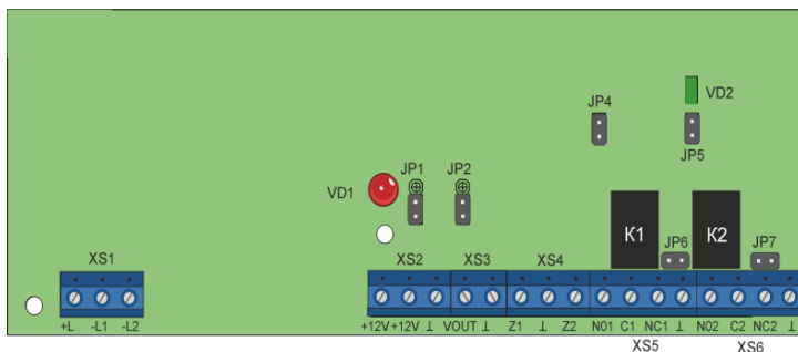
Рис. 2 Внешний вид платы МШ4-2
