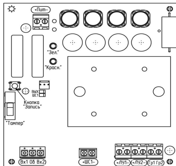
Рисунок 2 (а) - Танго-ОП/ГР20
