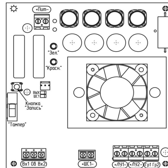
Рисунок 2 (б) - Танго-ОП/ГР100
