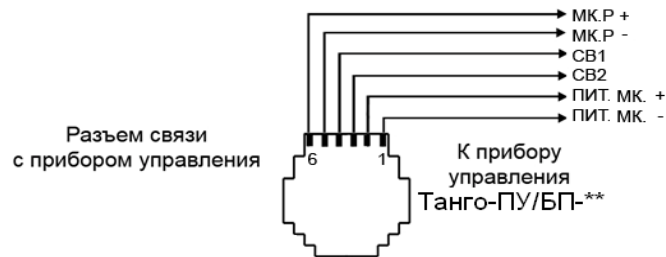
Рисунок 1 – Разъем подключения прибора управления .
