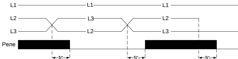
Рисунок 6. Контроль порядка чередования и обрыва фаз
