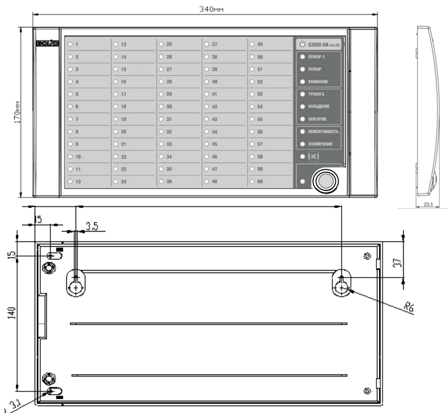
Рисунок 1. Внешний вид, габаритные и установочные размеры блока
