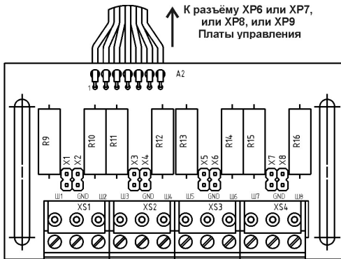
Рисунок 3 - Внешний вид модуля МШ-08
