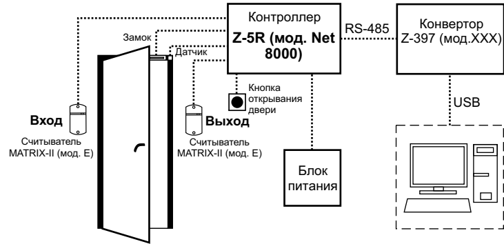
Рис.1 Схема СКУД с контроллером Z-5R (мод. Net 8000)
