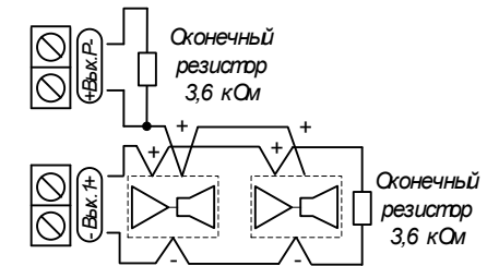
Рисунок 3.2 Схема подключения без контроля линии речевого сигнала
