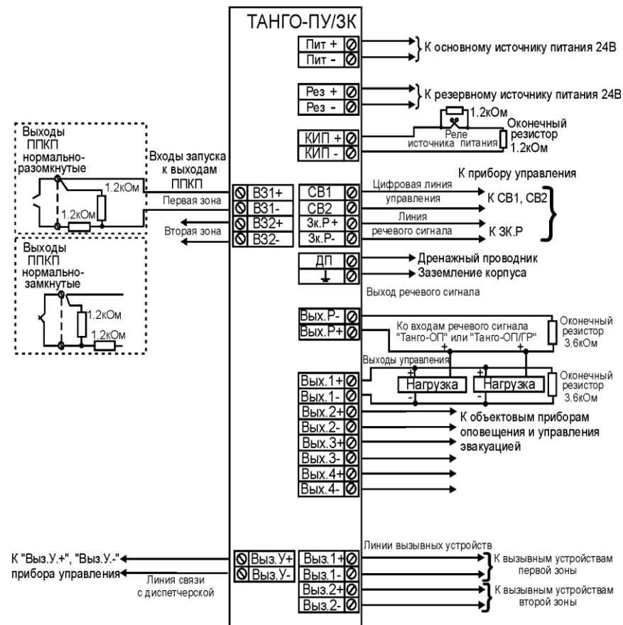
Рисунок 6 - Монтажная схема зонального коммутатора
