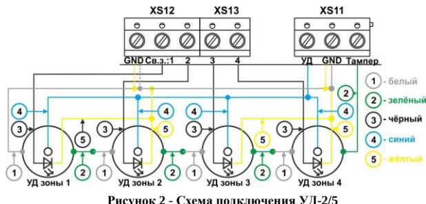
Рисунок 2 - Схема подключения УД-2/5
