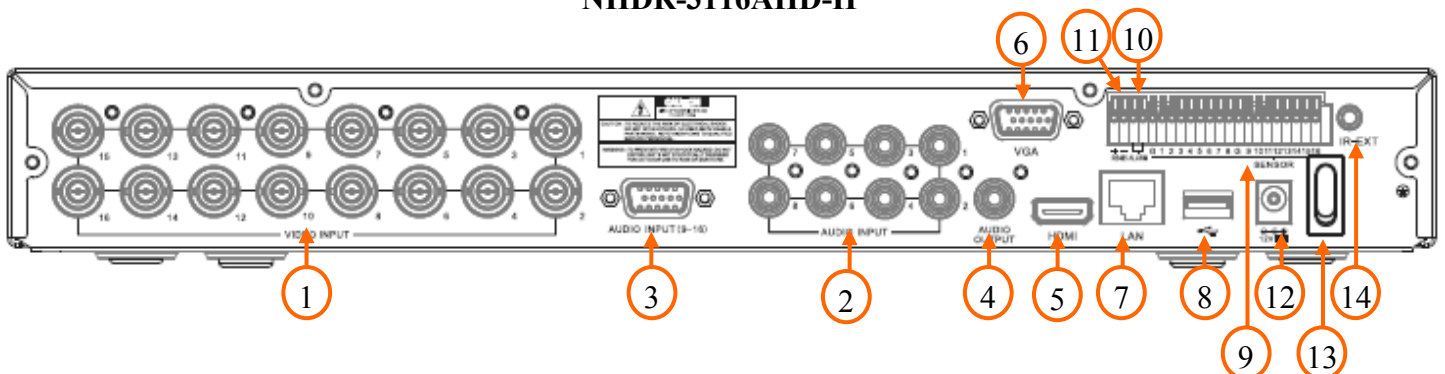
NHDR-3116AHD-II
