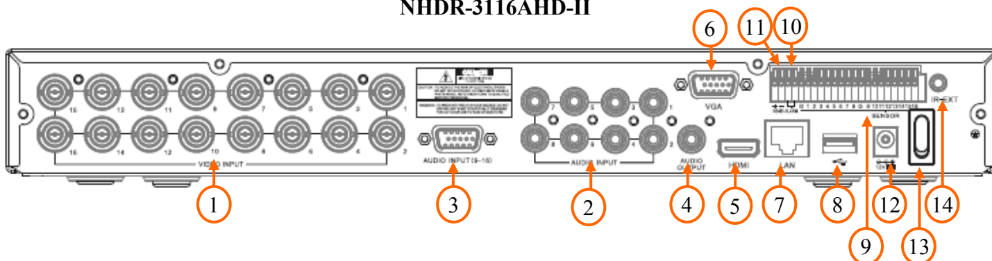
NHDR-3116AHD-II
